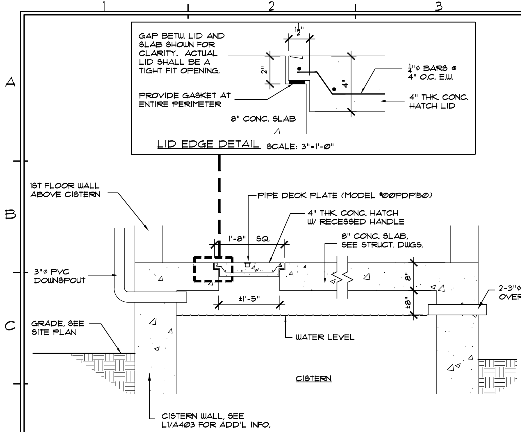
D1 CISTERN MANHOLE DETAIL
